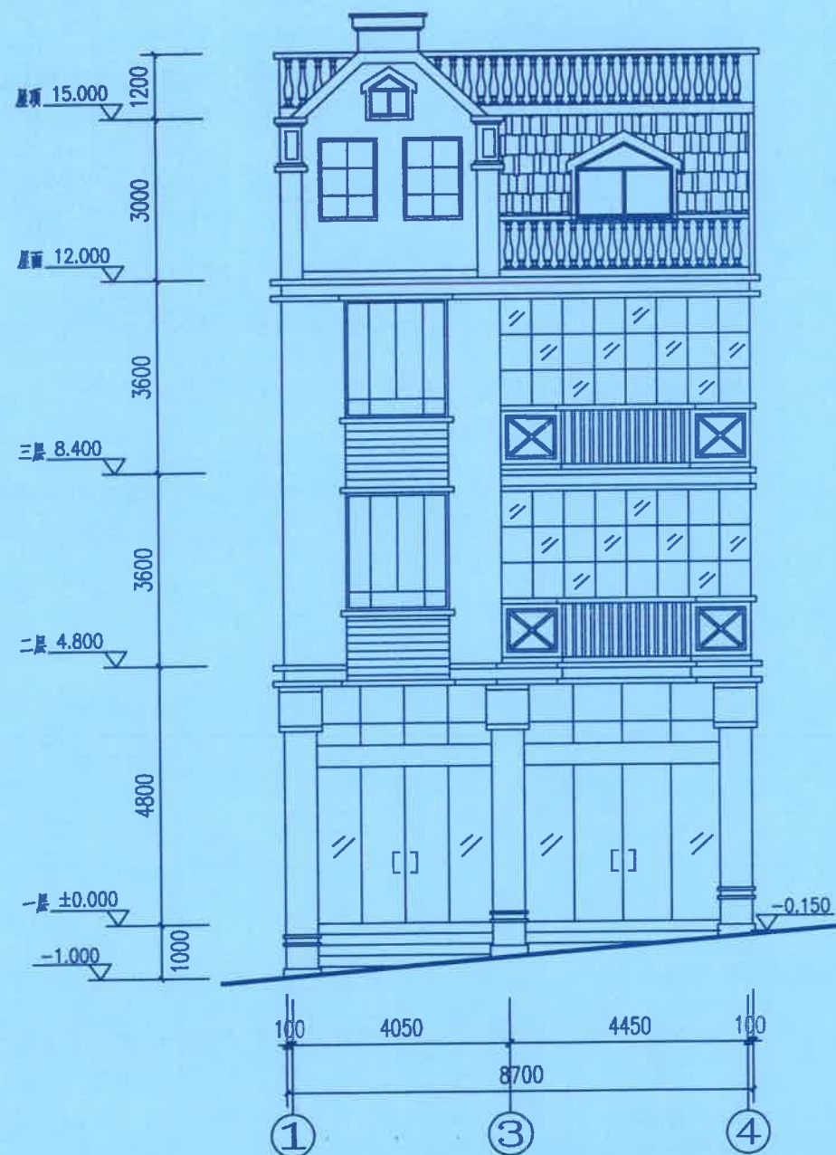
①-④ 轴立面图(变更前) 1:100
